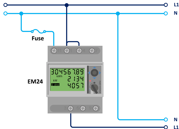
EM24 connecté comme un compteur de réseau monophasé à fonction unique
