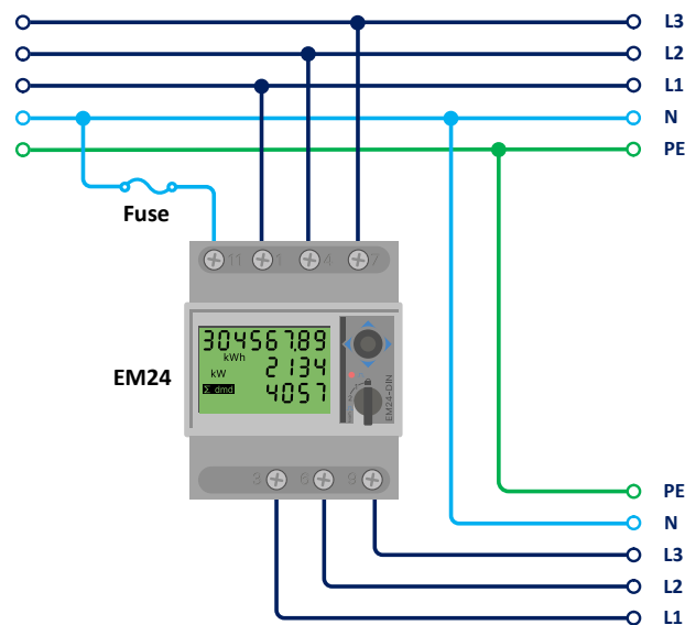
Câblage triphasé EM24
